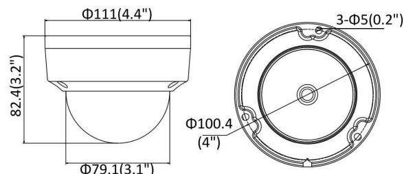
Kamera AVILINK-IP180
