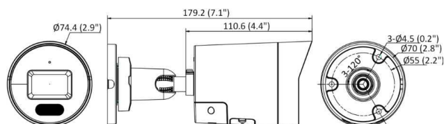
Wymiary kamery AVILINK-IP260
